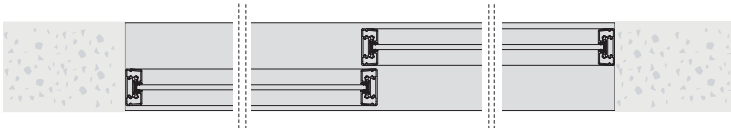
A SOFFITTO Ceiling - Au plafond -De techo
